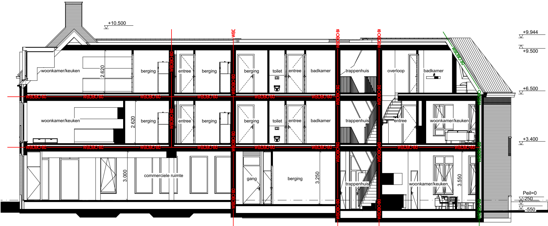
Doorsnede A-A
