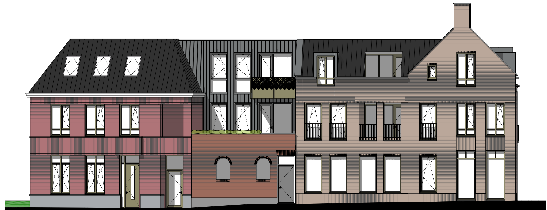
Linkergevel
