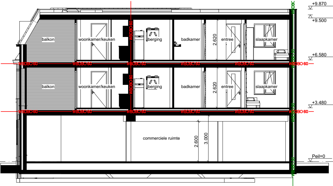
Doorsnede B-B
