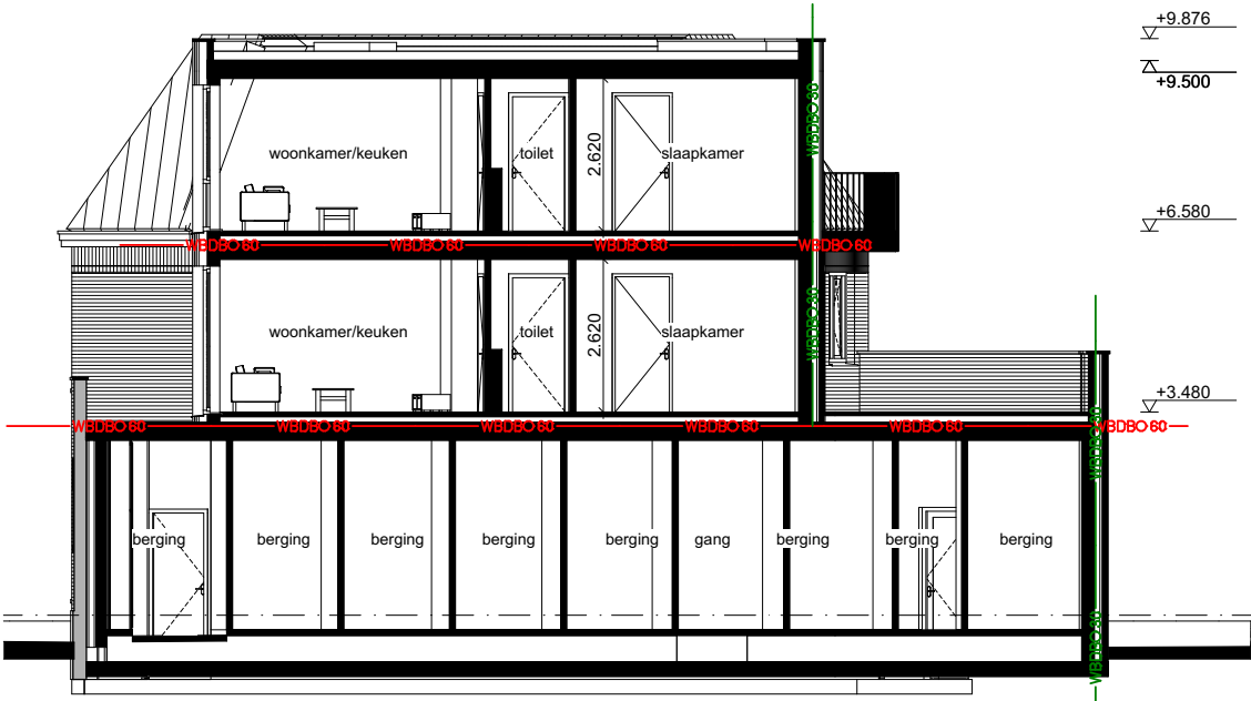
Doorsnede C-C
