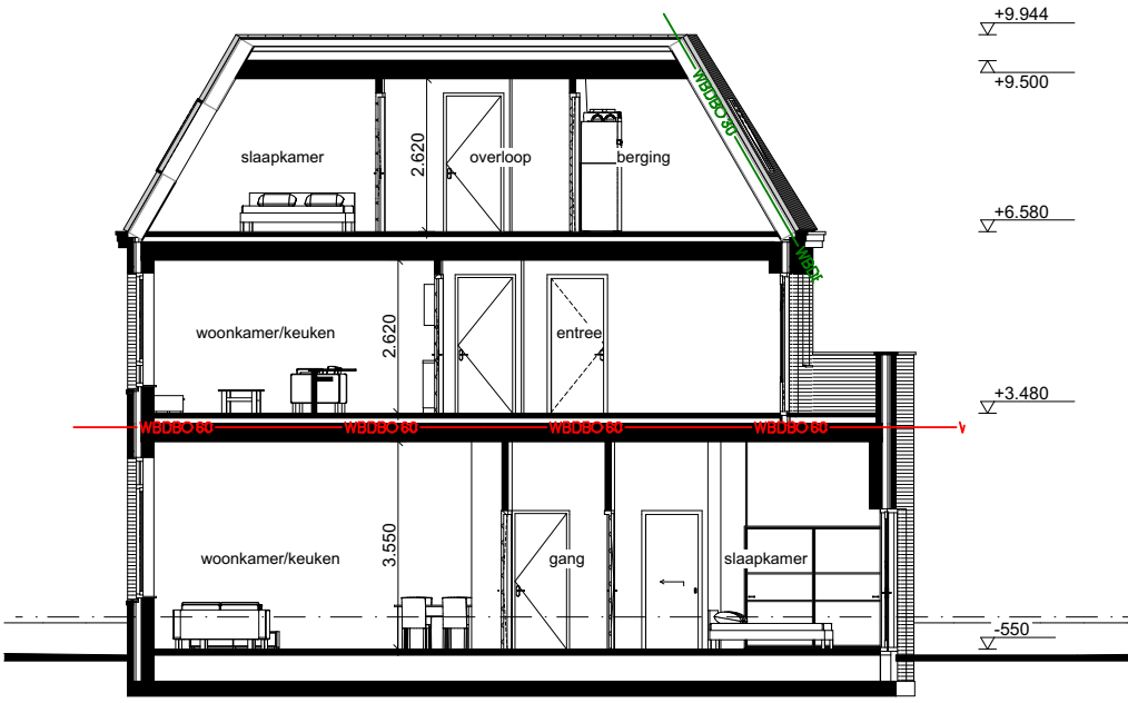
Doorsnede D-D
